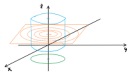
Abb. 12: Koordinatenlinien bzw. -flächen der Zylinderkoordinaten (r, \varphi, z) .
