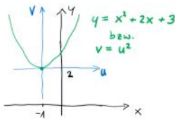
Abb. 2: Quadratische Funktion in zwei kartesischen Koordinatensystemen
