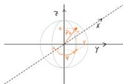
Abb. 13: Darstellung der Kugelkoordinaten (r, \vartheta, \varphi) .
