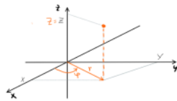
Abb. 11: Darstellung der Zylinderkoordinaten (r, \varphi, z) .
